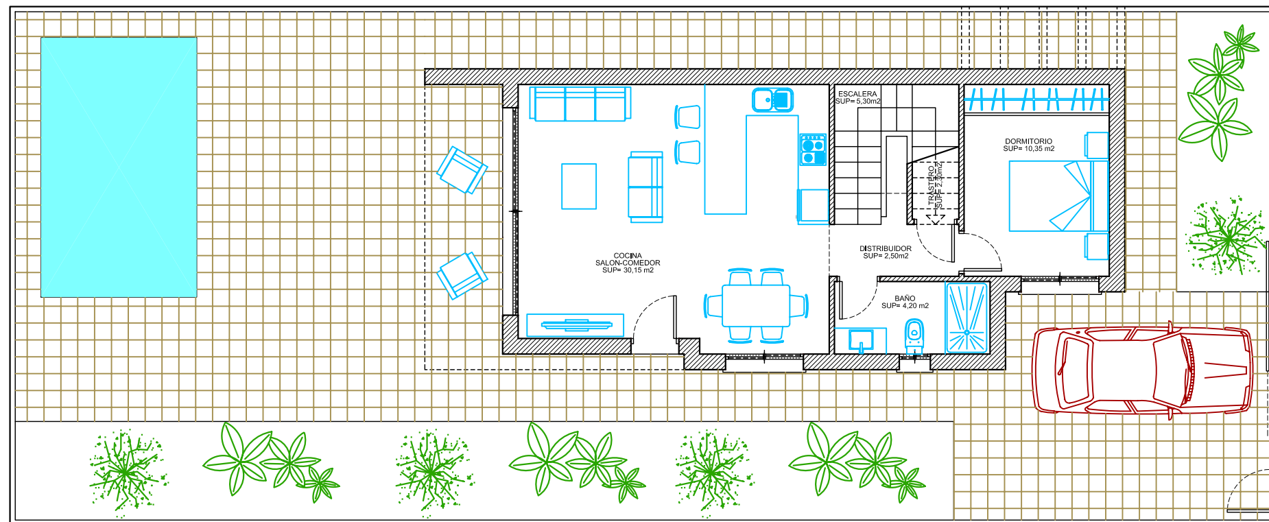
PLANTA BAJA
